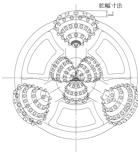
カッタービット寸法表 (トリコン・スポーク)
